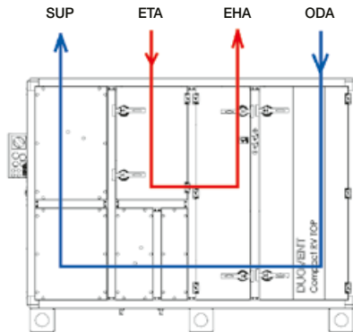
Right neck position „R“
