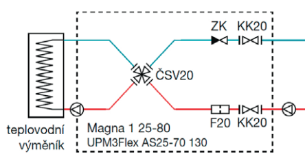
ESU čtyřcestný směšovací uzel Kv 6,3 - 16
