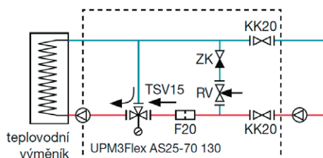
ESU třícestný směšovací uzel Kv 0,6 - 4,0
