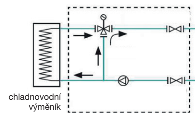
ESUCH rozdělovací uzel
