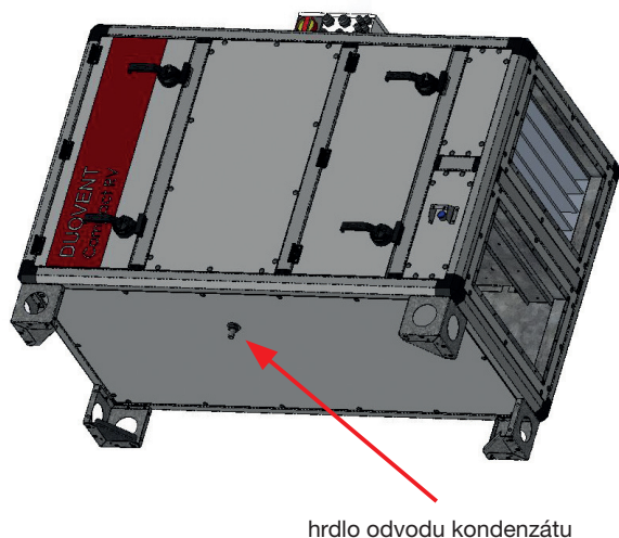
hrdlo odvodu kondenzátu
