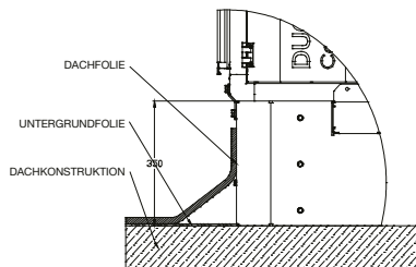
Einbaubeispiel des Untergestellrahmens ROOFPACK-B in die Dachkonstruktion
