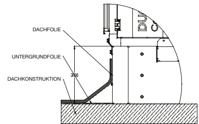
Einbaubeispiel des Untergestellrahmens ROOFPACK-B in die Dachkonstruktion
