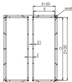
DETAIL DES VERBINDUNGSSUTZENS INTEGRIERT IN DER WANDPLATTE
