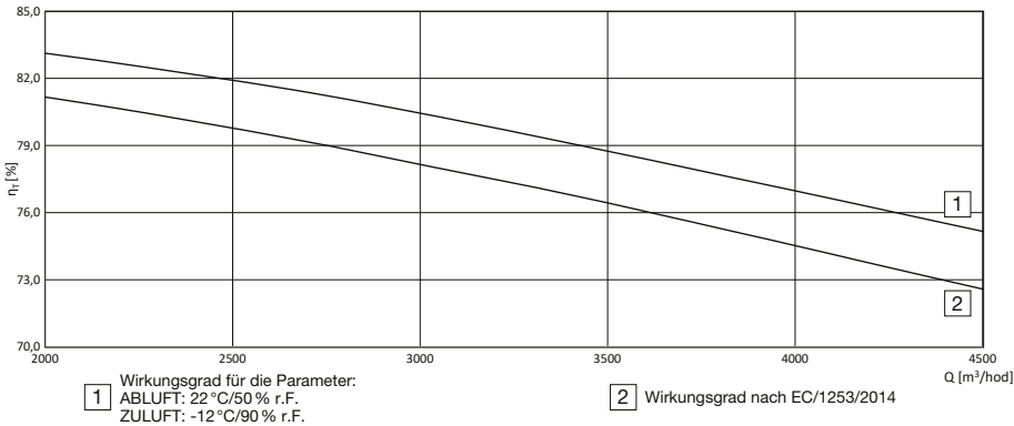
DUOVENT® COMPACT RV 4200 TOP – WÄRME-Wirkungsgrad der Rückgewinnung
