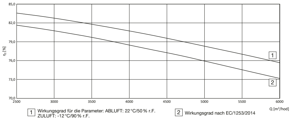
DUOVENT® COMPACT RV 6000 TOP – WÄRME-Wirkungsgrad der Rückgewinnung
