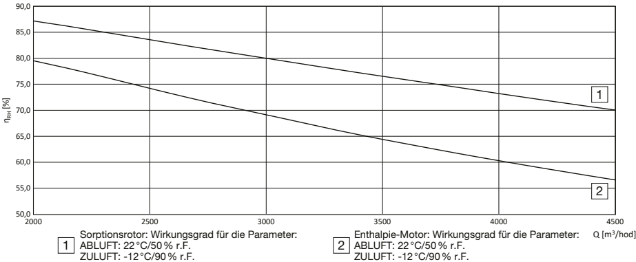
DUOVENT® COMPACT RV 4200 TOP – FEUCHTIGKEITS-Wirkungsgrad der Rückgewinnung
