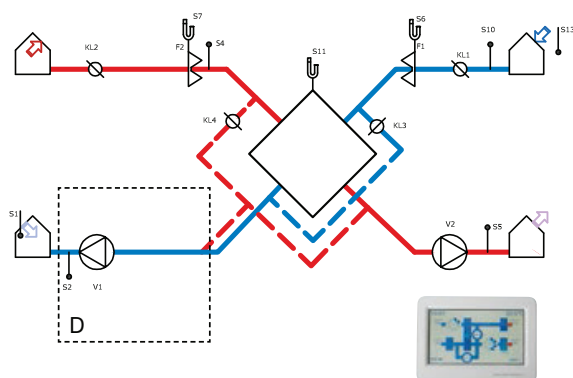
deskový výměník
