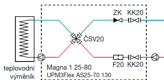
ESU čtyřcestný směšovací uzel Kv 6,3 - 16
